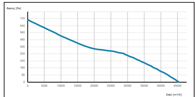
K-CAXI 900-5-40
