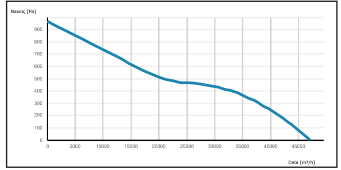
K-CAXI 900-8-40
