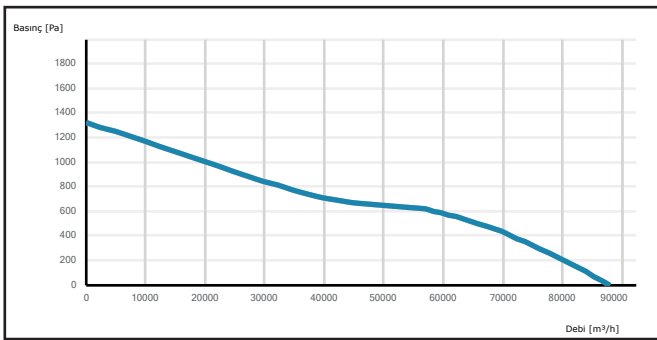
K-CAXI 1120-8-40
