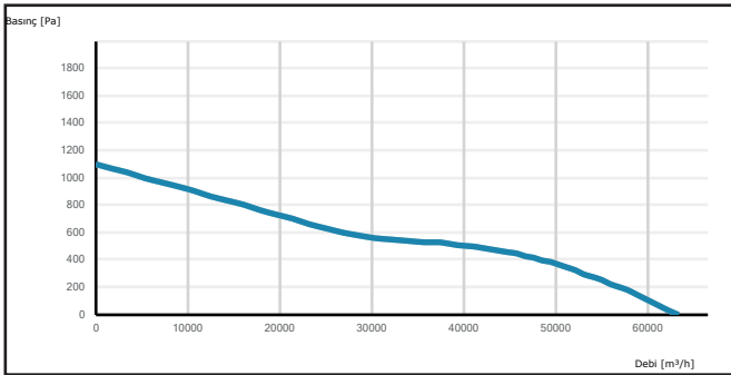
K-CAXI 1000-8-40
