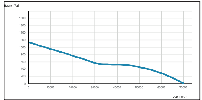
K-CAXI 1000-8-45
