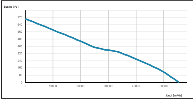
K-CAXI 1000-5-40
