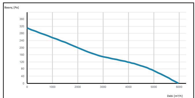
K-TAXI 500-5-25
