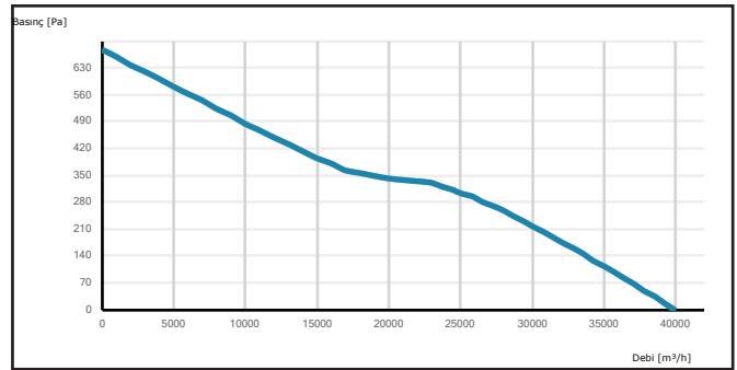
K-TAXI 900-5-35
