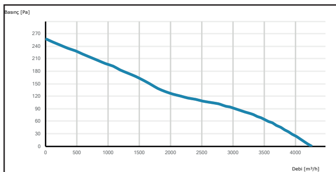
K-TAXI 450-5-25
